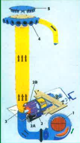
Sistema neumático. Pneumatic distributor. Distributeur pneumatique.
