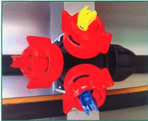
Portaboquillas Trijet con antigoteo y tres boquillas.
