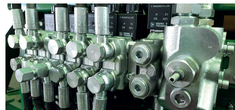
Mando electrohidráulico con línea sensora LS. Commande électro-hydraulique avec ligne de capteurs LS. Electro-hydraulic control with LS sensor line.
