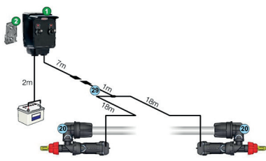
Boquillas punta eléctricas. Buses à pointe électrique. Electric tip nozzles.
