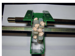
Distribuidor para semillas muy grandes (opción).
