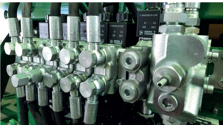
Mando electrohidráulico con línea sensora LS. Commande électro-hydraulique avec ligne de capteurs LS. Electro-hydraulic control with LS sensor line.
