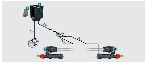
Kit boquillas eléctricas punta + caja 2 vías. Kit buses eléctricas + boîte à 2 voies. Electric nozzles kit + 2-way box.
