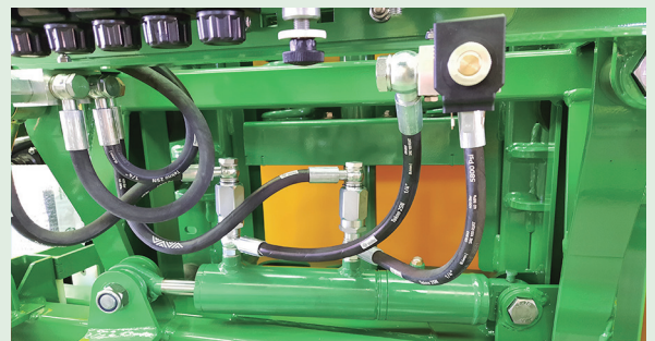
Bloqueo Hidráulico + Nivelación. Blocage hydraulique + Nivellement. Hydraulic Locking + Levelling.
